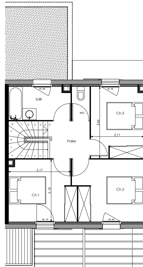
ETAGE
